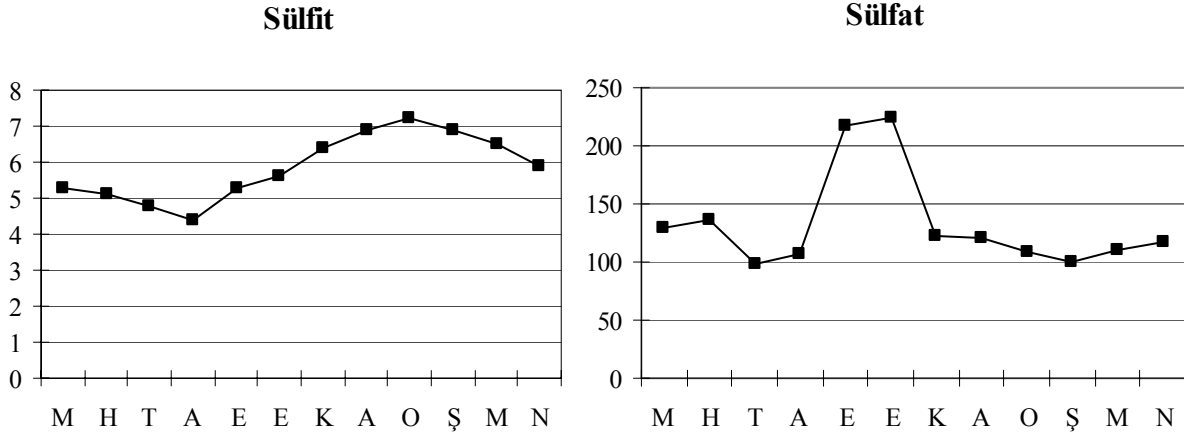
Şekil 8. Aylık Sülfid ( \text{Na}_2\text{SO}_3 ) ve Sülfat ( \text{SO}_4^{2-} ) (mg/L) seviyeleri
